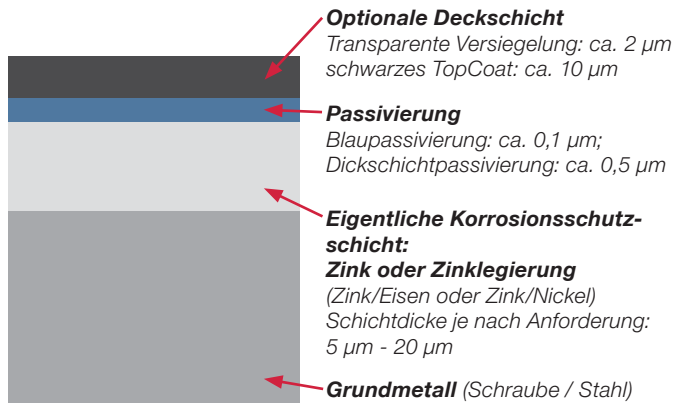
Prinzipieller Aufbau einer galvanischen Beschichtung
