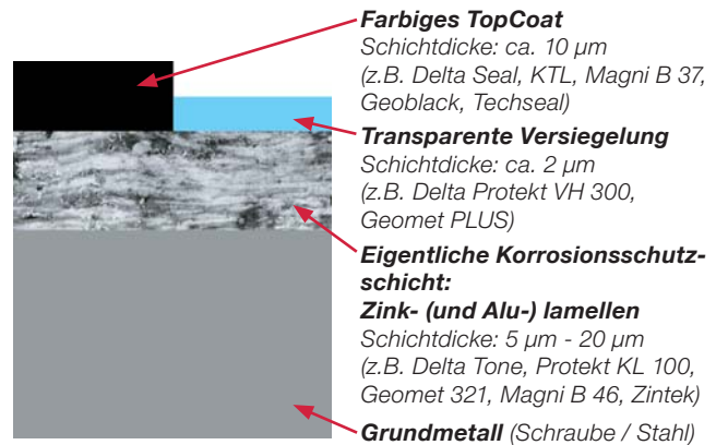
Prinzipieller Aufbau eines Zinklamellen-Systems
